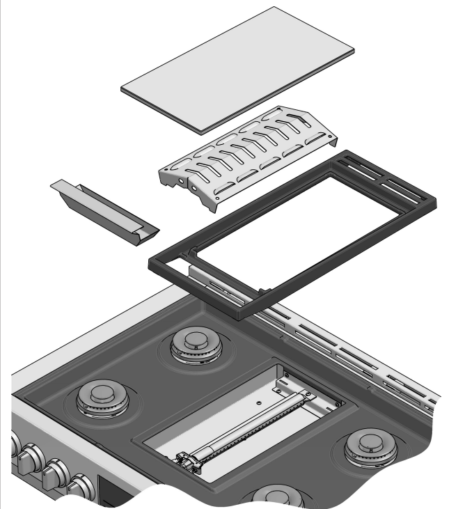
VUE ÉCLATÉE DU GRIL-BRÛLEUR
