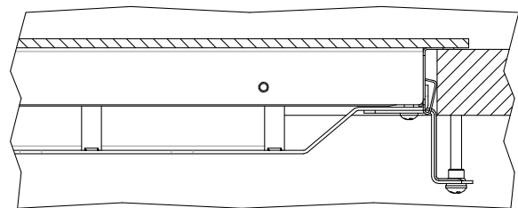
POSITION DER DICHTUNG BEI DER VERSION SEMIFILTOP
