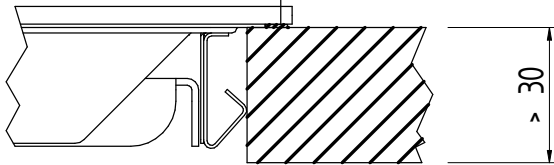
POSITION DER DICHTUNG BEI DER VERSION SEMIFILTOP
