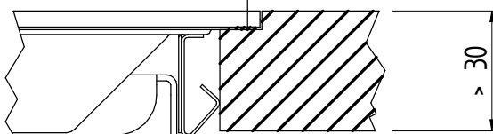
POSITION DER DICHTUNG BEI DER VERSION FILTOP (bündig)
